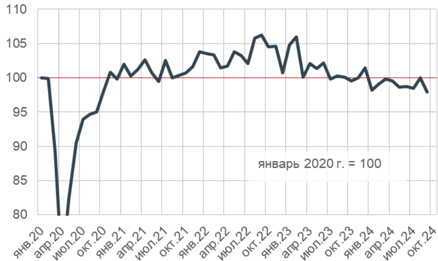
Промшленное производство
