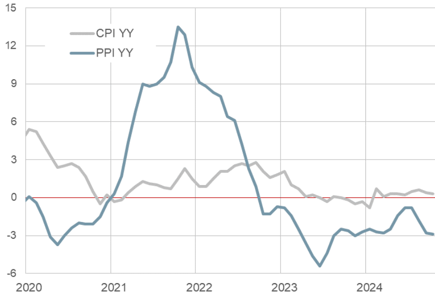
Инфляция, % г/г
