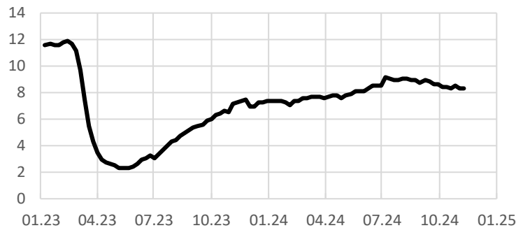
ИПЦ (справочно)
